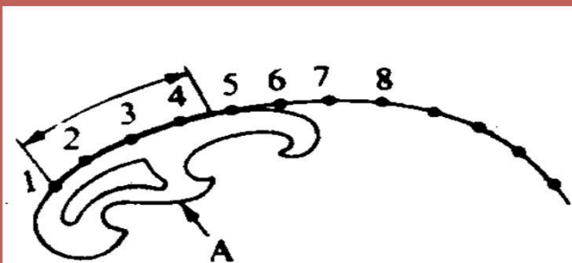
Gb. 3.9 Mal lengkungan.
