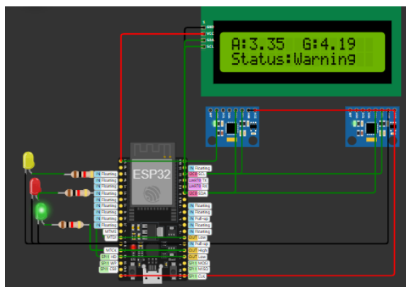
Gambar 2. Simulasi Wokwi Dengan Keluaran Gyros
