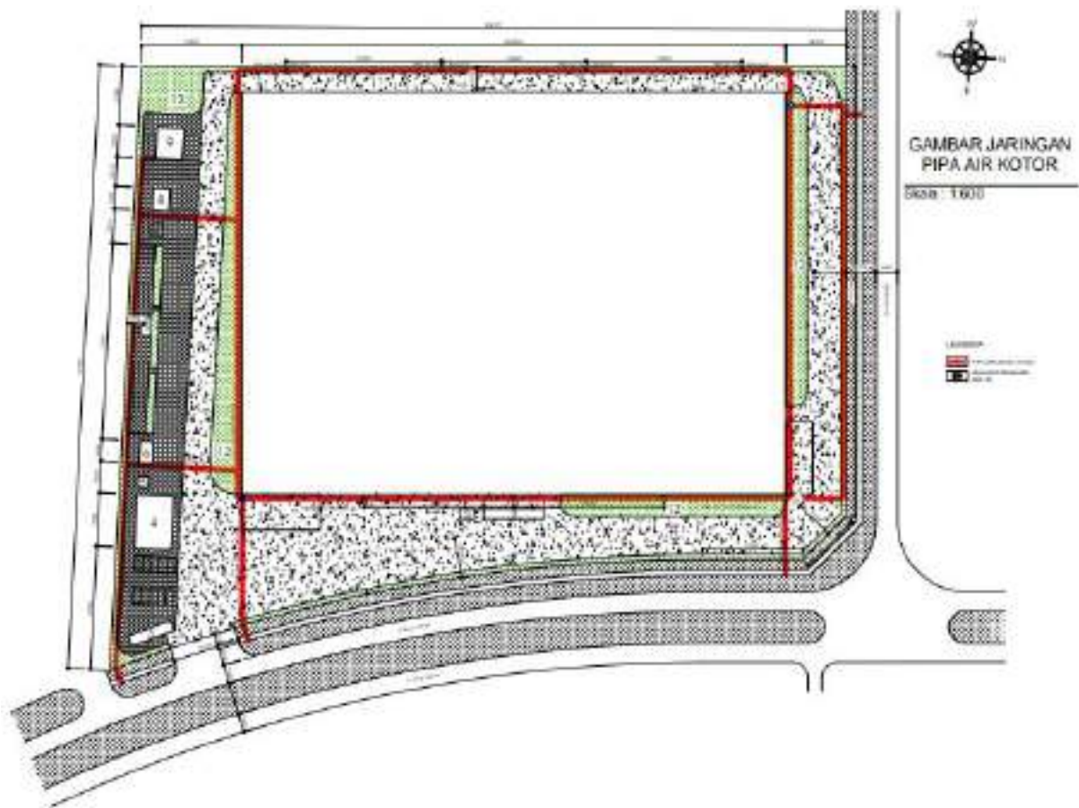
Gambar 4. 28 Detail instalasi air kotor Sumber: Hasil Pengamatan di lokasi
