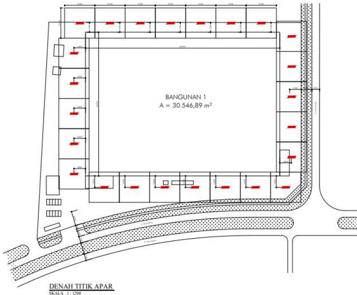
Gambar 4. 29 Detail denah titik lokasi APAR Sumber: Hasil Analisa di Lokasi Kegiatan
