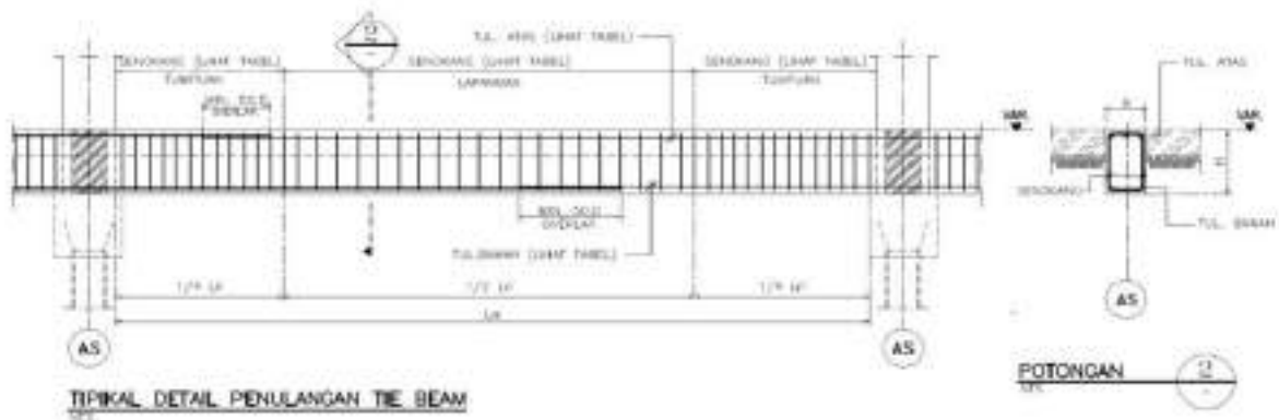
Gambar 4. 16 Penulangan tie beam Sumber: Hasil Analisa di Lokasi Kegiatan
