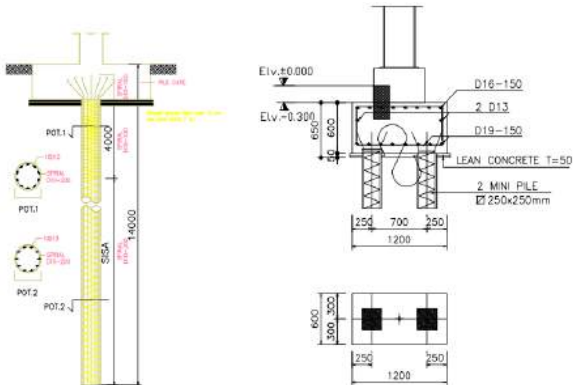
Gambar 4. 15 Detail Bore Pile Sumber: Hasil Analisa di Lokasi Kegiatan
