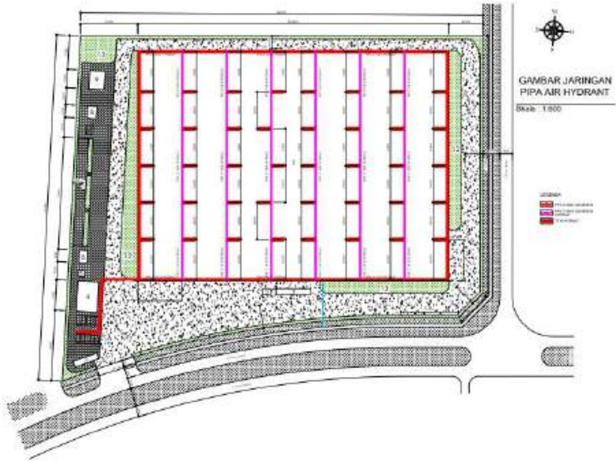
Gambar 4. 30 Detail denah titik lokasi Hydrant Sumber: Hasil Analisa di Lokasi Kegiatan
