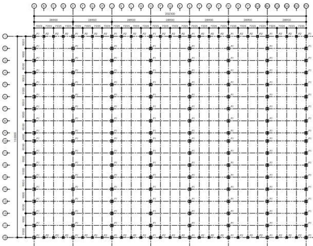
Gambar 4. 13 Denah titik pondasi Sumber: Hasil Analisa di Lokasi Kegiatan
