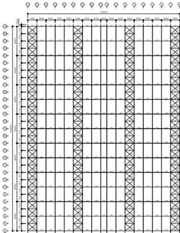
Gambar 4. 19 Detail Rangka Atap Sumber: Hasil Analisa di Lokasi Kegiatan
