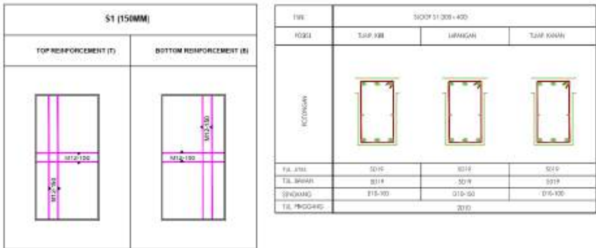
Gambar 4. 17 Detail plat lantai dan Dimensi Pembesian Sumber: Hasil Analisa di Lokasi Kegiatan
