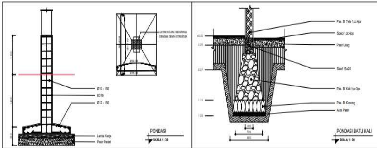
DENAH PONDASI DAN SLOOF SKALA 1 : 500
