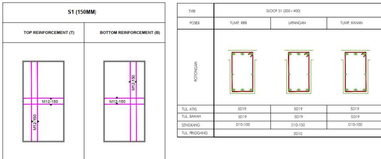
Gambar 4. 17 Detail plat lantai dan Dimensi Pembesian Sumber: Hasil Analisa
