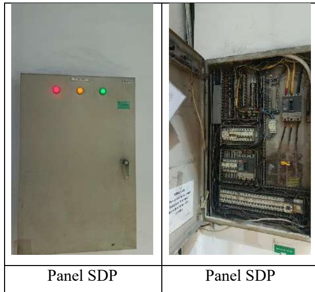
Gambar 4. 25 Kondisi Panel SDP Sumber: Hasil Analisa
