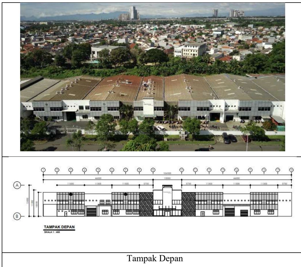
Gambar 4. 1 Tampak Bangunan PT. Voestalpine Bohler Welding Asia Pasific Sumber: Hasil Analisa Dokumen Pribadi
