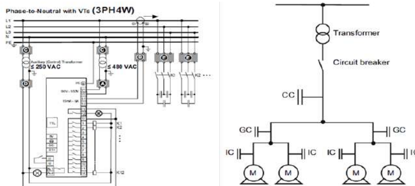
Gambar 4. 26 Gambar Lay-Out Kapasitor Bank Sumber: Hasil Analisa
