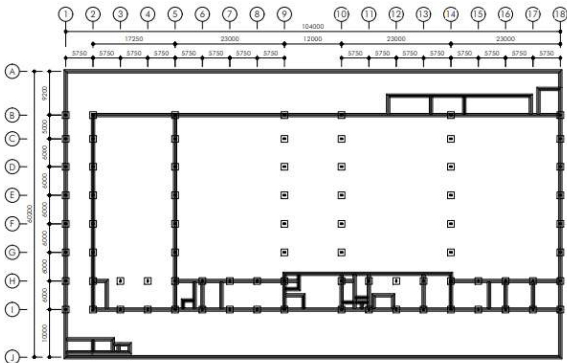
Gambar 4. 13 Denah titik fondasi Sumber: Hasil Analisa
