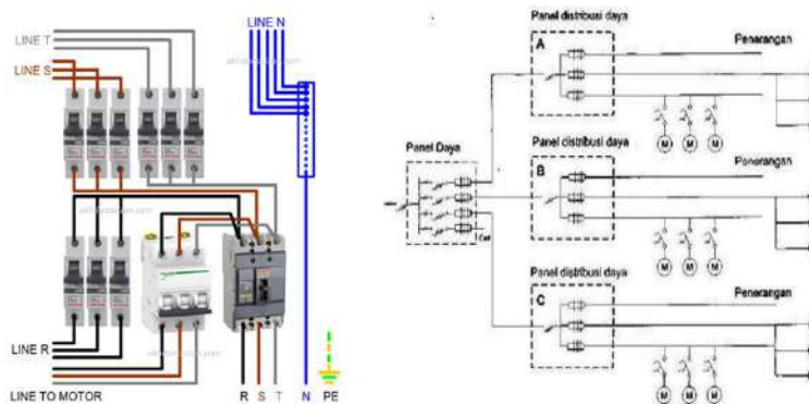
Gambar 4. 28 Gambar Lay-Out Panel SDP Sumber: Hasil Analisa
