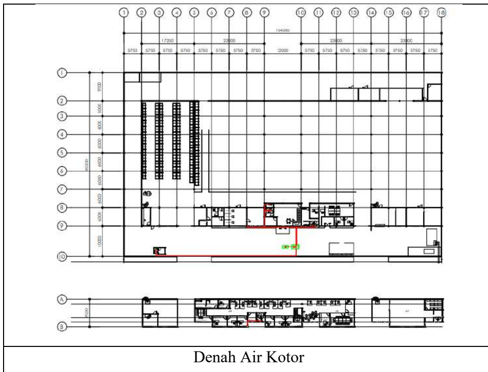
Gambar 4. 36 Detail instalasi air kotor Sumber: Hasil Analisa
