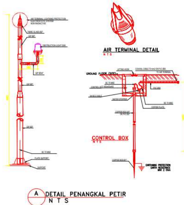
Gambar 4. 31 Sistem penangkal petir & Grounding Sumber: Hasil Analisa
