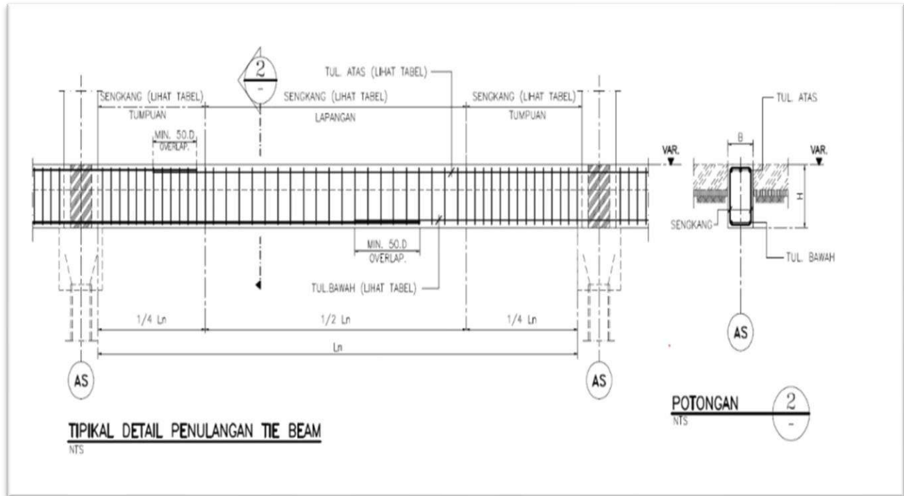
Gambar 4. 16 Penulangan tie beam Sumber: Hasil Analisa
