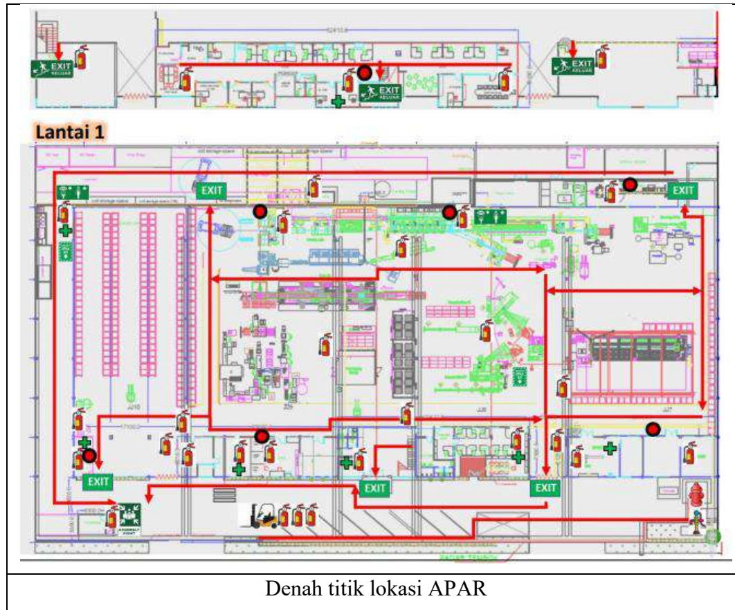
Gambar 4. 38 Detail denah titik lokasi APAR Sumber: Hasil Analisa
