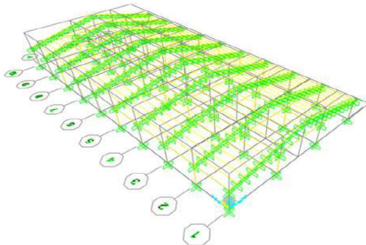
Gambar 4. 18 Analisa pembebanan dan pemodelan struktur bangunan Sumber: Hasil Analisa
