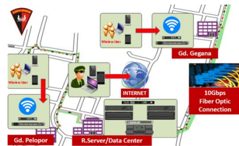
Gambar 2: Ilustrasi Jaringan Komunikasi SIAB
