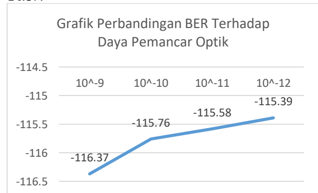
Gambar 13: Grafik Perbandingan BER Terhadap Daya Pemancar Optik
