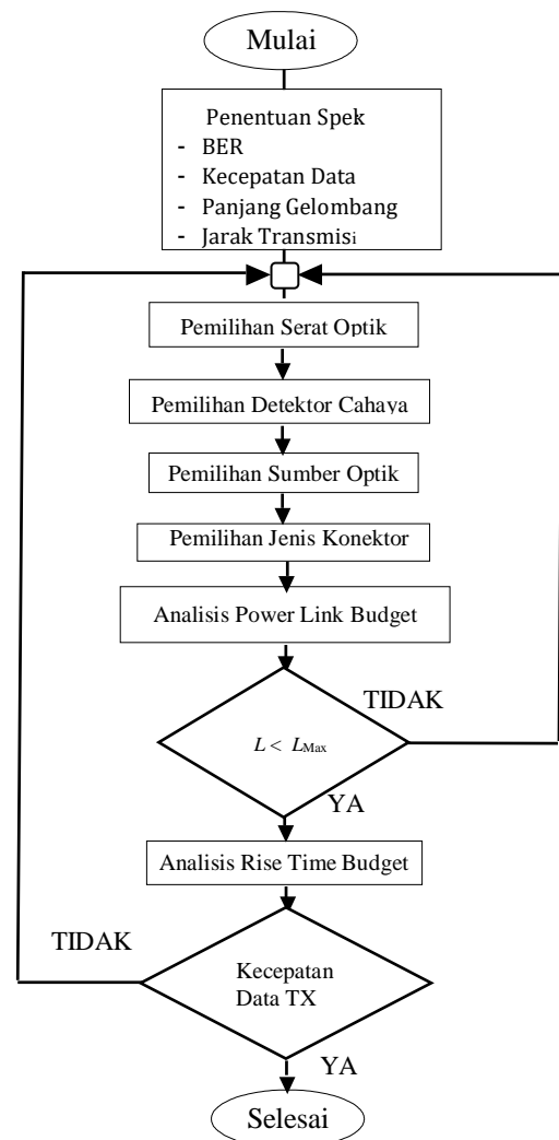
Gambar 5: Flow Chart Perencanaan Jaringan Komunikasi SIAB
