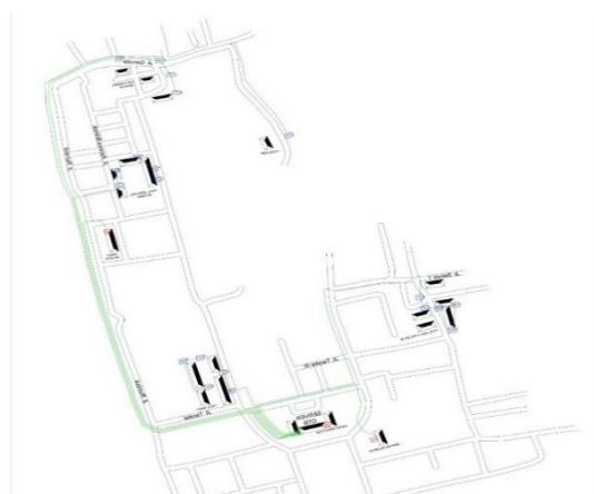
Gambar 4: Jalur Kabel Serat Optik Jaringan Komunikasi SIAB
