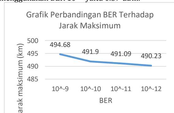
Gambar 14: Grafik Perbandingan BER Terhadap Jarak Maksimum
