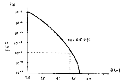
Gambar 8: Grafik 0,5 erfc
