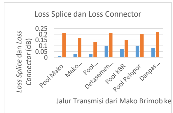
Gambar 10: Grafik Loss Splice dan Loss Connector Jalur Transmisi Mako Brimob
