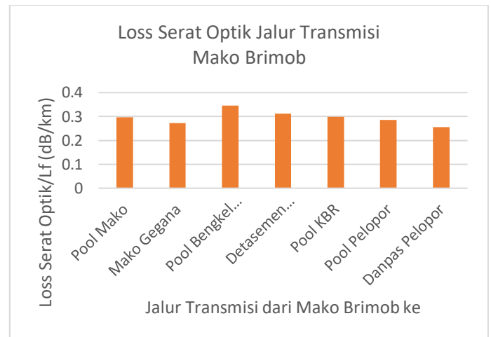
Gambar 9: Grafik Loss Serat Optik Jalur Transmisi Mako Brimob
