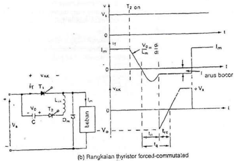
Gambar 4-10 Karakteristik turn-off
