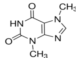
Teobromin
