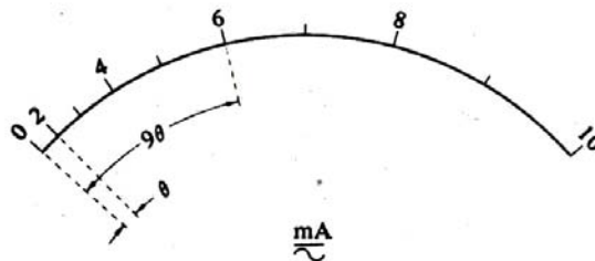
Gambar 6 Skala suatu alat ukur jenis thermokopel
