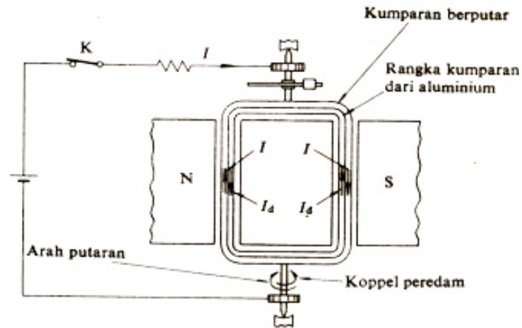
Gambar 4 : mekanisme peredaman alat ukur kumparan putar
