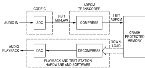
Gambar 3.8 Proses Uji Coba SSCVR Sinyal Suara Memakai PATS
