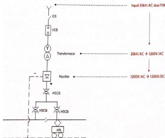
Gambar 2.2 Single Land Diagram Sederhana Sistem Elektrifikasi DC.
