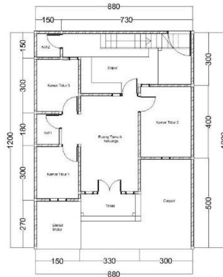
Gambar 5. Denah Rumah Sumber: Dokumentasi Pribadi
