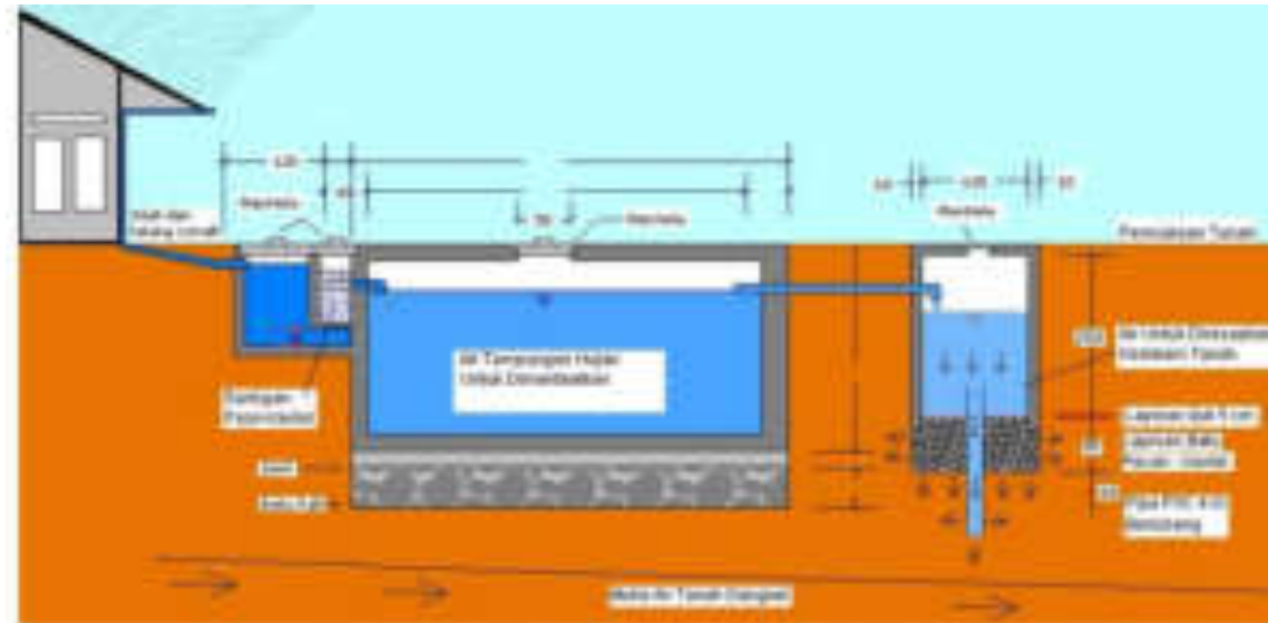
Gambar Sistem Penampungan Air Hujan (SPAH) dan Sumur Resapan (SRES)
