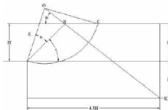
Gambar 2.16. Lokasi pusat busur longsor kritis pada tanah kohesif
