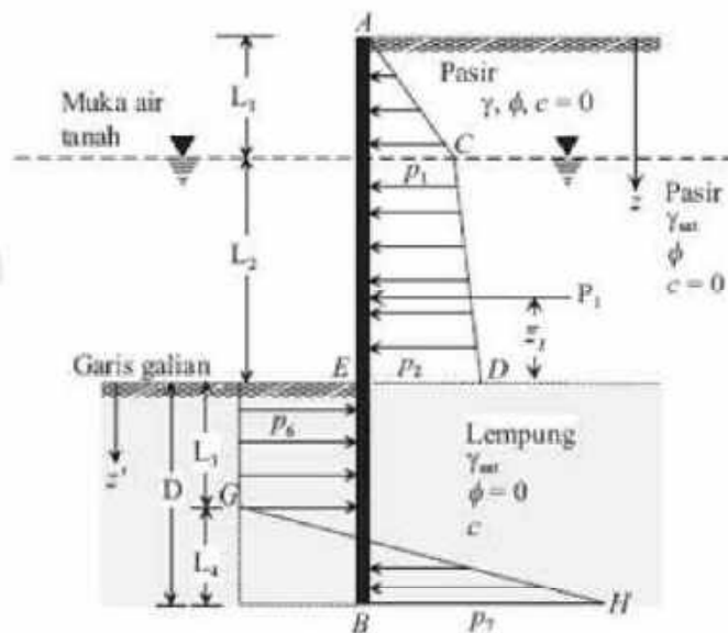
Gambar 2.24 Tiang turap cantilever tertanam pada lapisan lempung
