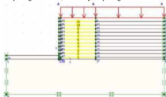
Gambar 2.27 Gambar contoh pembebanan dalam Plaxis
