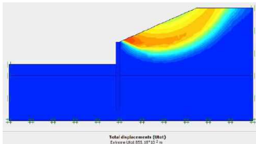
Gambar 4.25 Pemancangan bore pile dengan analisa Plaxis 8.2 (total displacement)
