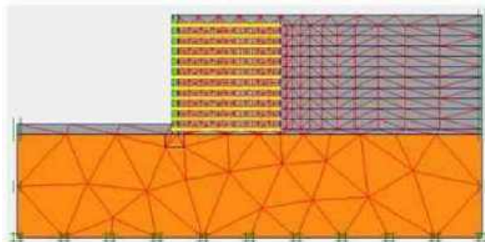
Gambar 2.34 Contoh setelah meng-klik generate mesh
