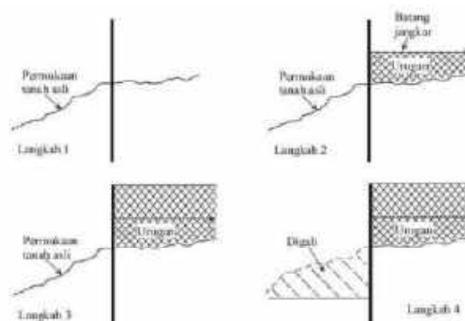
Gambar 2.21 Langkah-langkah konstruksi untuk struktur galian
