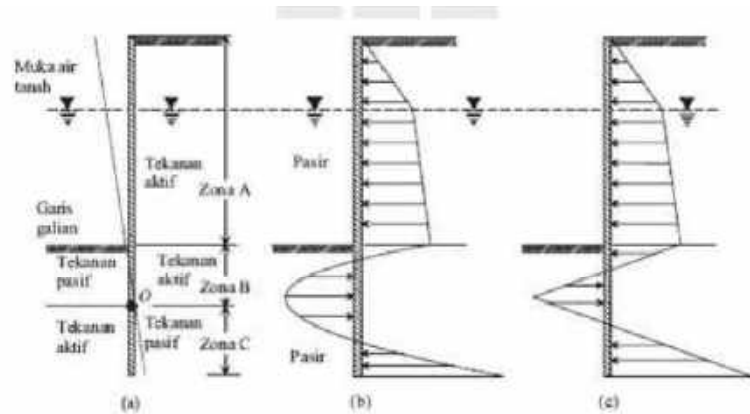
Gambar 2.22 Tiang turap cantilever tertanam pada pasir
