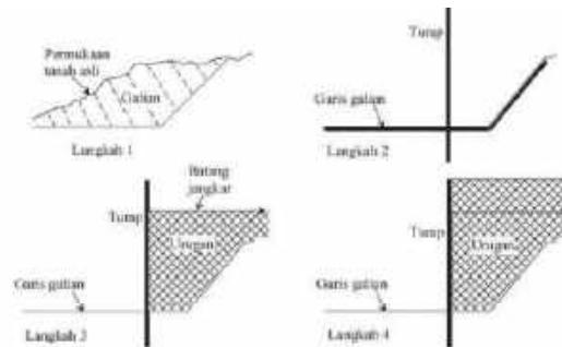
Gambar 2.20 Langkah-langkah konstruksi untuk struktur urugan
