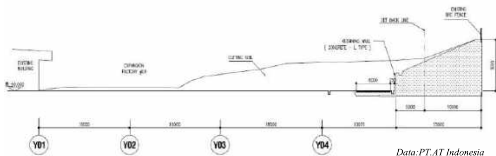
Gambar 3.3 Penampang perencanaan cantilever wall
