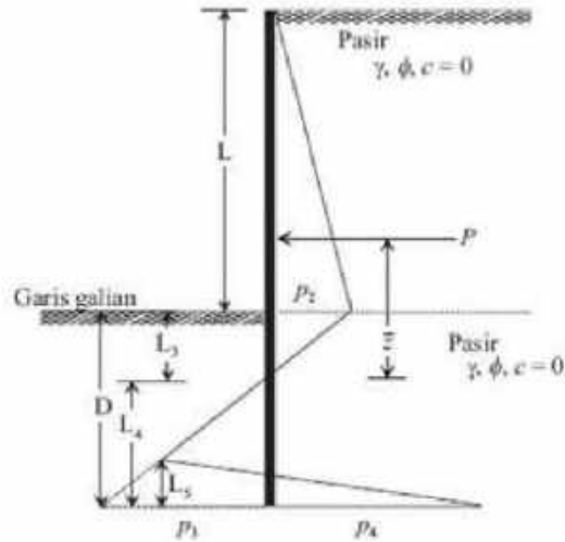
Gambar 2.23 Turap cantilever tertanam pada pasir tanpa muka air
