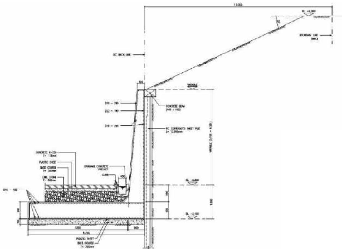
Gambar 3.4 Detail perencanaan cantilever wall
