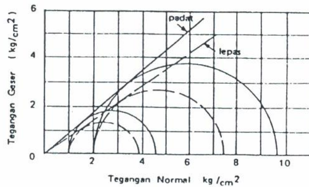
LINGKARAN-LINGKARAN MOHR
