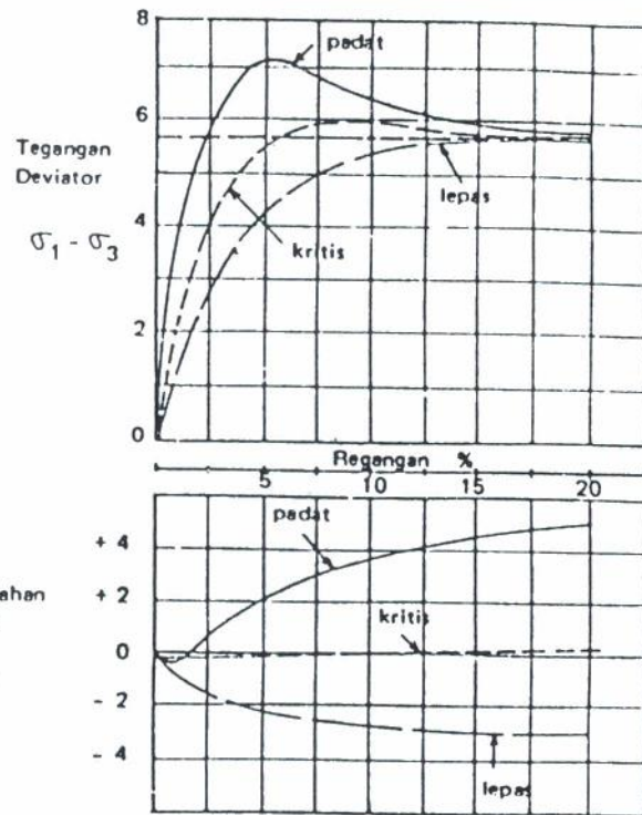
GRAFIK TEGANGAN DEVIATOR DAN PERUBAHAN ISI TERHADAP REGANGAN
