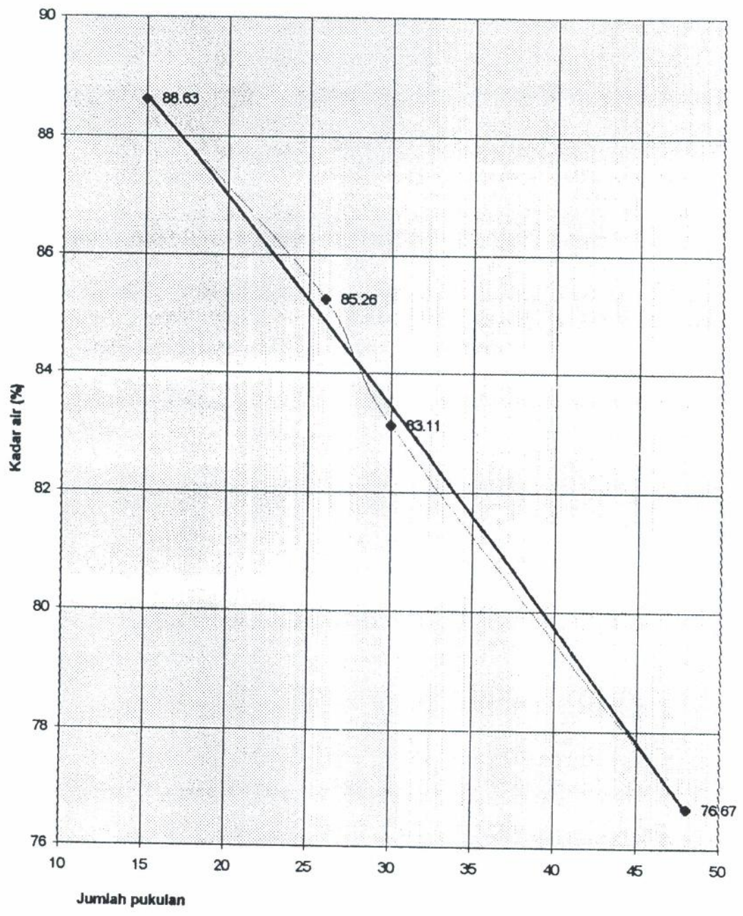
Gambar 4.1.1. Hubungan jumlah pukulan dan kadar air pada liquid limit tanah asli
