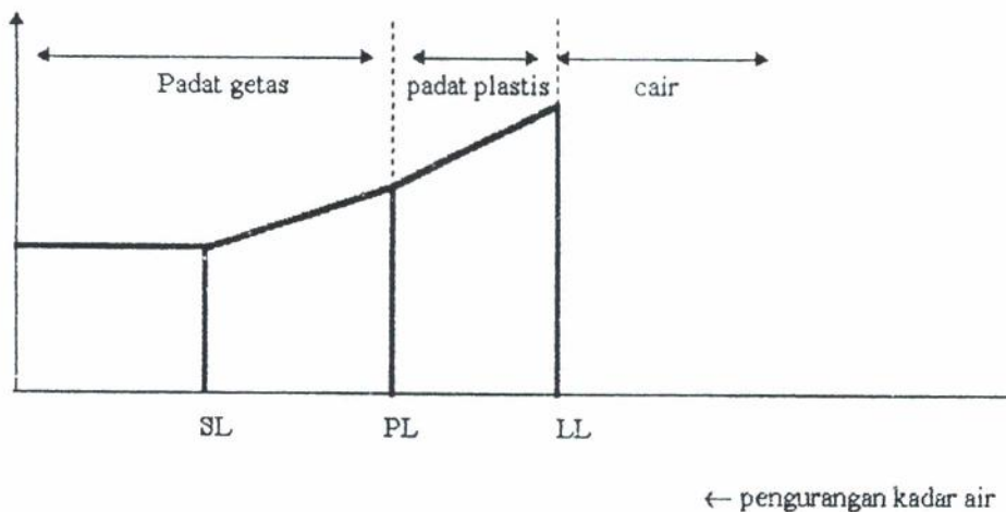
Gambar 2 : Variasi volume dan kadar air pada kedudukan batas cair, batas plastis dan batas susutnya.
