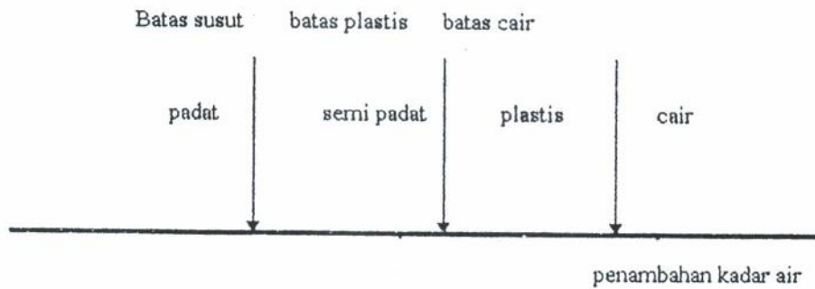
Gambar I : Batas-batas Atterberg
