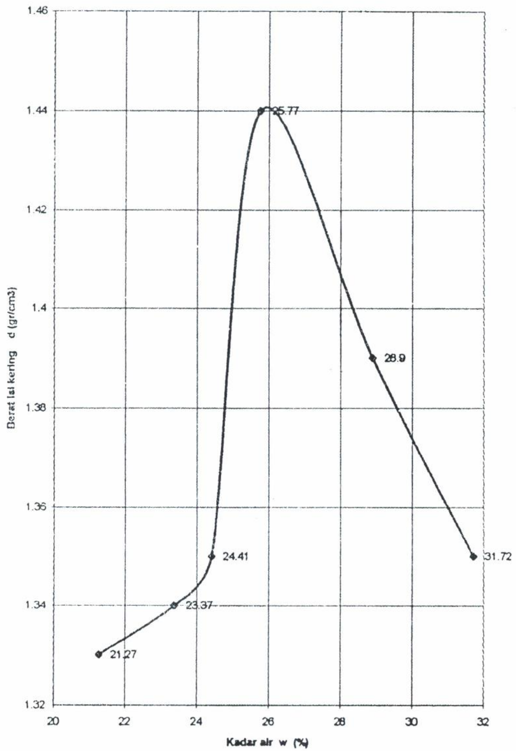
Gambar 4.1.1.1. Hasil pemadatan tanah asli
