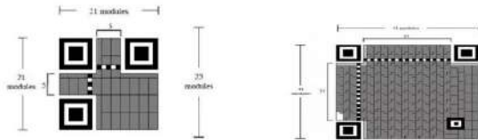
Gambar 2.7. QR code versi 1 (kiri) dan versi 2 (kanan)
