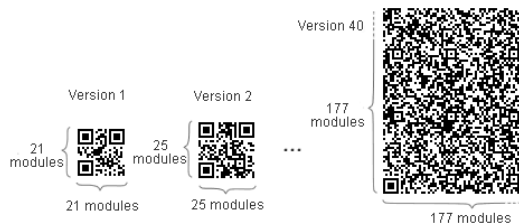
Gambar 2.8. Versi QR code
