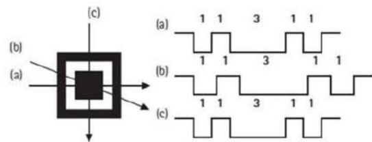
Gambar 2.4. Salah satu finding pattern QR code.
