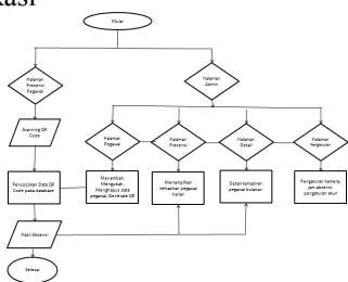
Gambar 3.2. Diagram alir aplikasi
