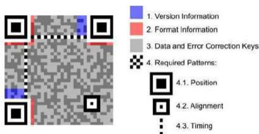
Gambar 2.3. Struktur QR code
