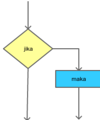
Gambar 5.1. Logika Percabangan
