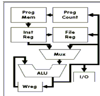
Gambar 5. Skema Mikroprosessor
